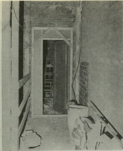
Estado actual de las obras en el exterior de nuestro piso. Los ladrillos que están en la parte izquierda sobre el suelo, cubren el hueco que dejó la bomba al caer al segundo piso.
