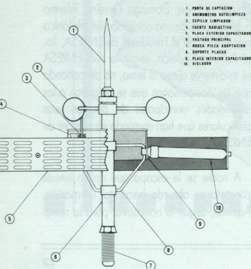
DETALLE DE UN PARARRAYOS RADIATIVO
