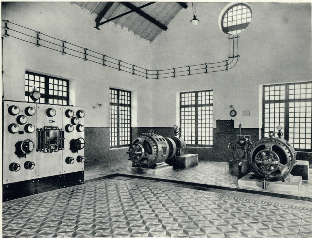
Sala de máquinas de la "Electra Aitzgorri". Potencia, 800 caballos.
