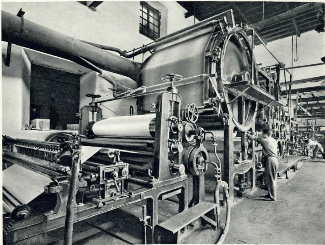
Máquina continua num. 1.
