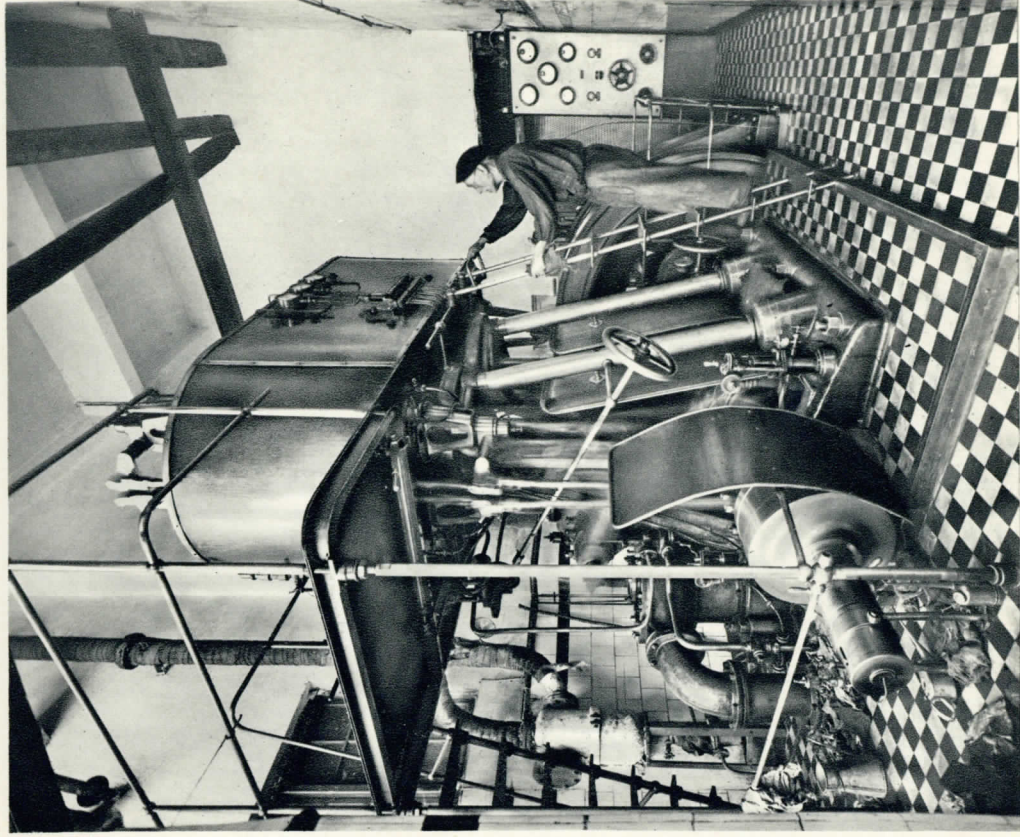
Máquina de vapor. Potencia, 400 caballos.
