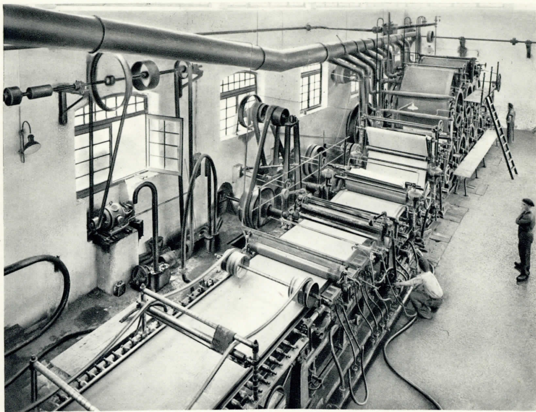
Máquina continua núm. 2.
