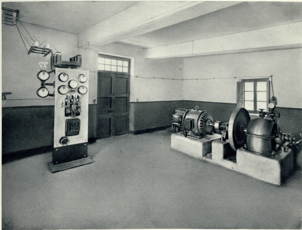
Interior de la Central Hidroeléctrica "San Adrián".
