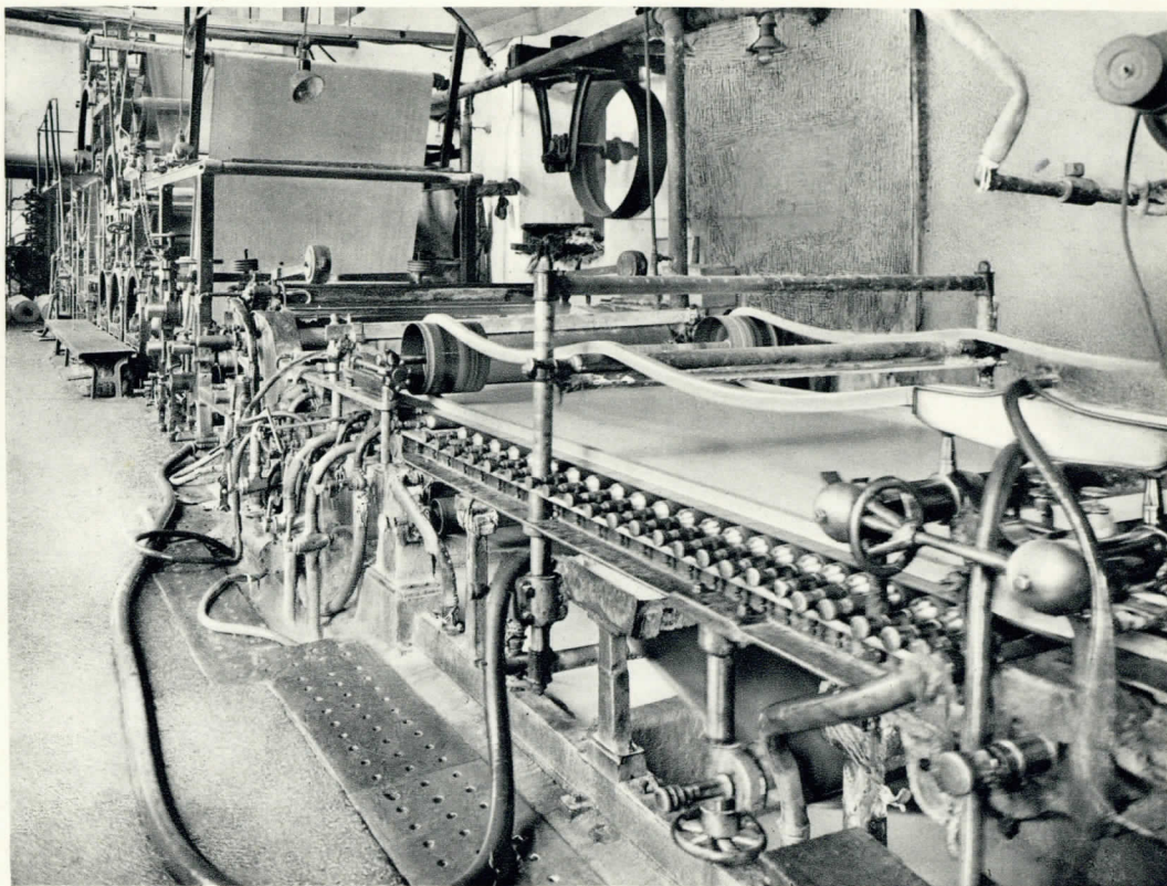
Máquina continua núm. 1.
